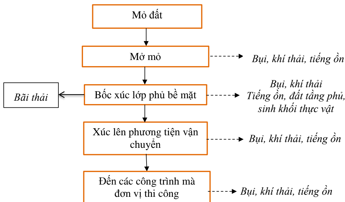
Hình 1.5: Quy trình khai thác mỏ đất
