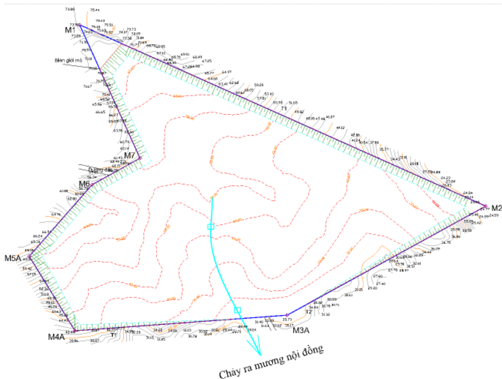
Hình 3.4: Sơ đồ rãnh thoát nước mưa
