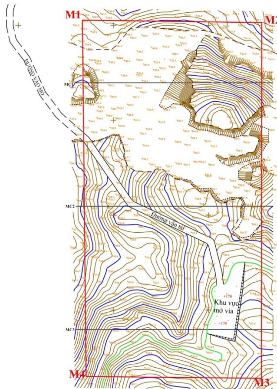
Hình 1.4: Sơ đồ mở vỉa
