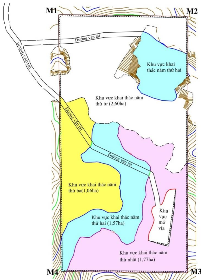
Hình 1.3: Sơ đồ khu vực khai thác từng năm
