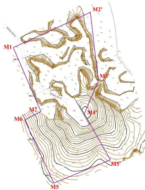
Hình 1.4: Sơ đồ mở vỉa
